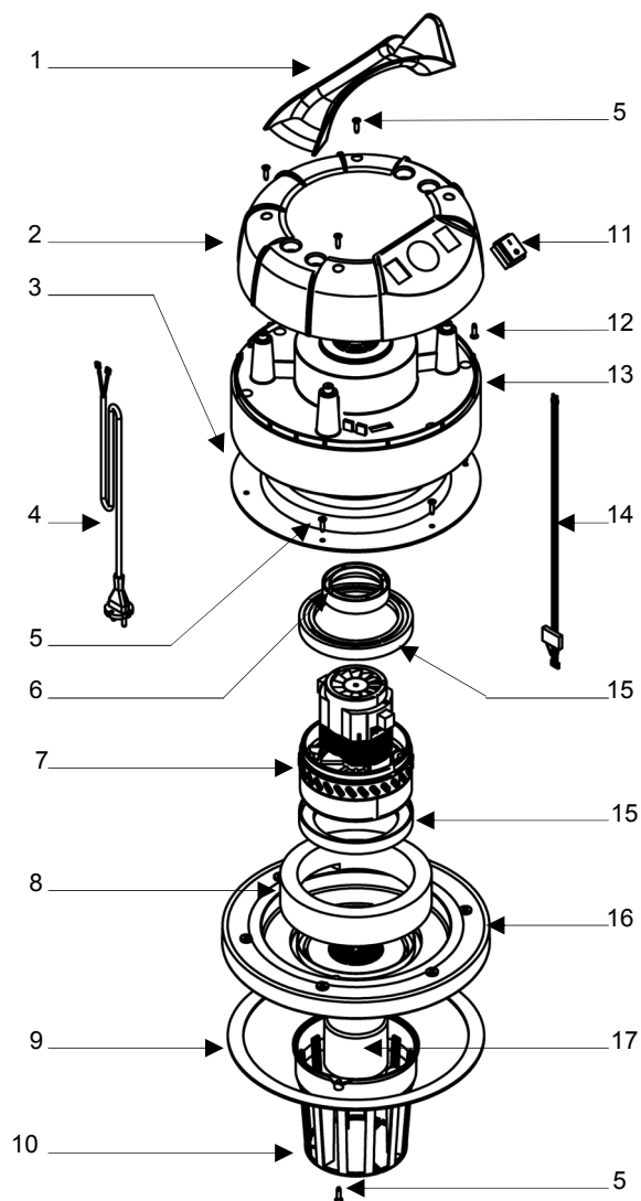
Complete motor head, Tête complète, Motorkopf kpl. Testa completa
